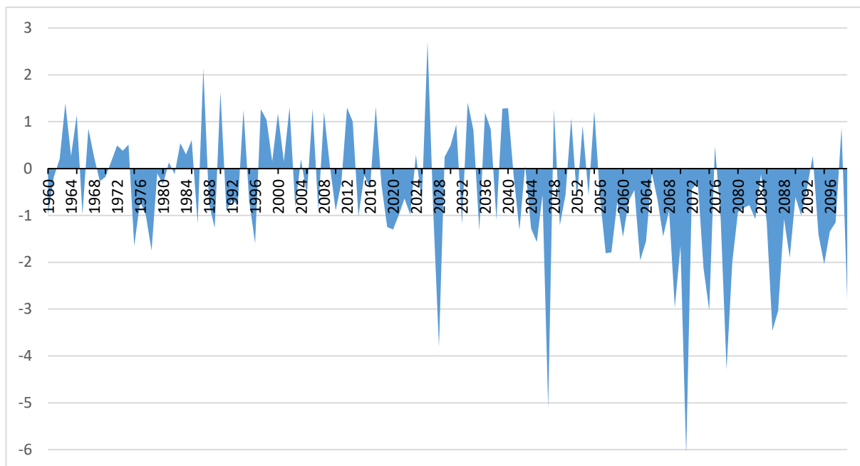
Figure 5 : Evolution de l'indicateur de sécheresse météorologique annuel moyen scénario A1B entre 1960 et 2100
