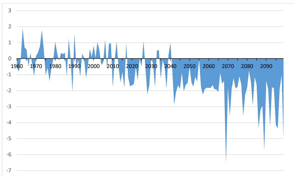
Figure 6 : Evolution de la sécheresse agricole annuelle moyenne depuis 1960 et prévision jusqu'à 2100 (scénario A1B)
