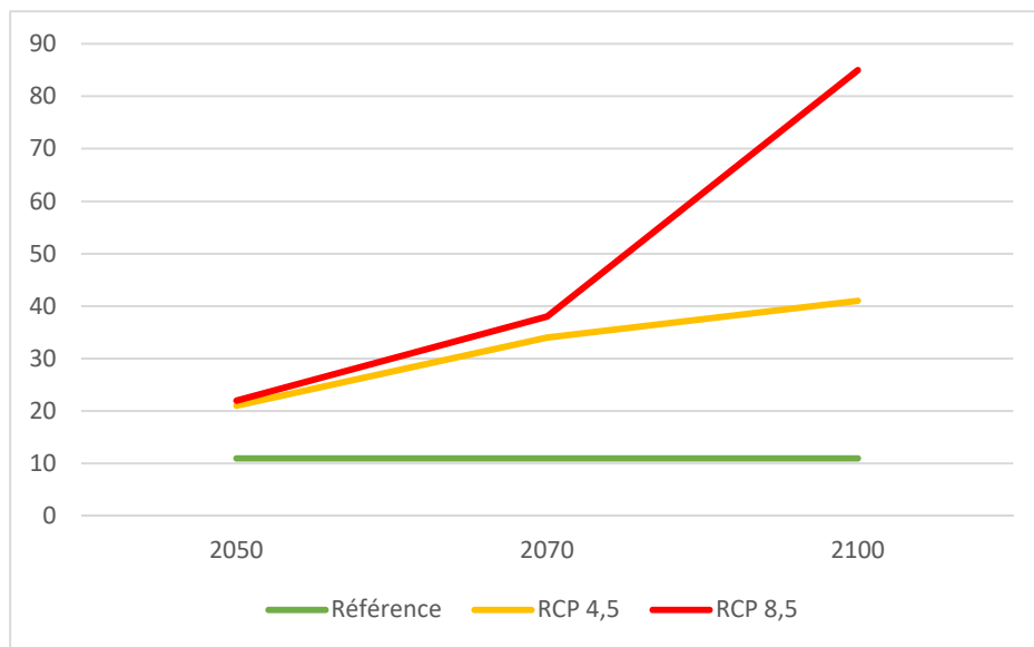
Figure 4 : Evolution du nombre moyen annuel de jours de vague de chaleur par RCP et par horizon
