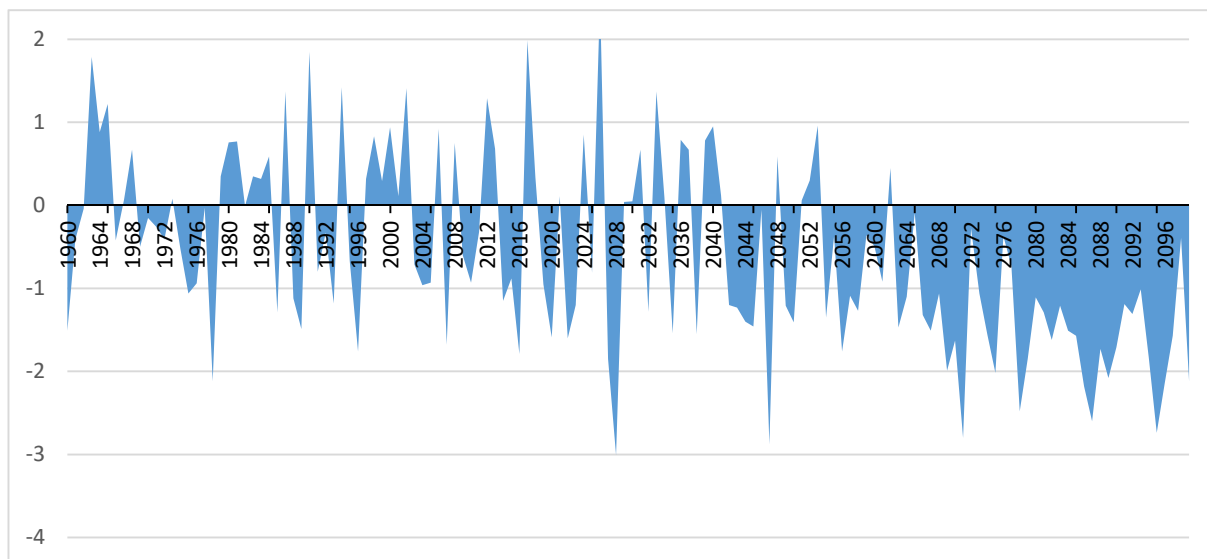
Figure 5 : Evolution de l'indicateur de sécheresse météorologique moyen annuel scénario A1B entre 1960 et 2100
